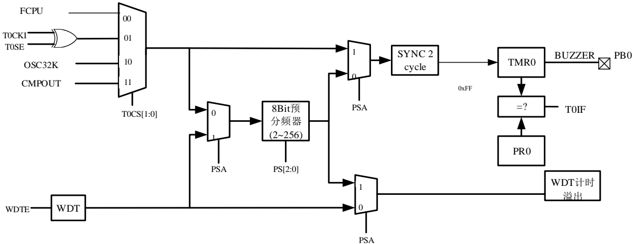
图 7.1.5: Timer0/WDT Prescaler 结构图
