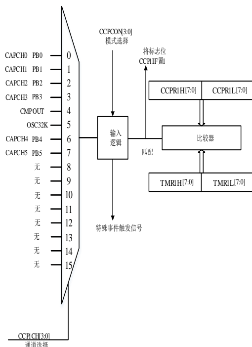
CCP1 捕捉模式工作原理图
