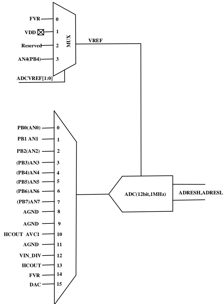
图 14.1 A/D 结构图
