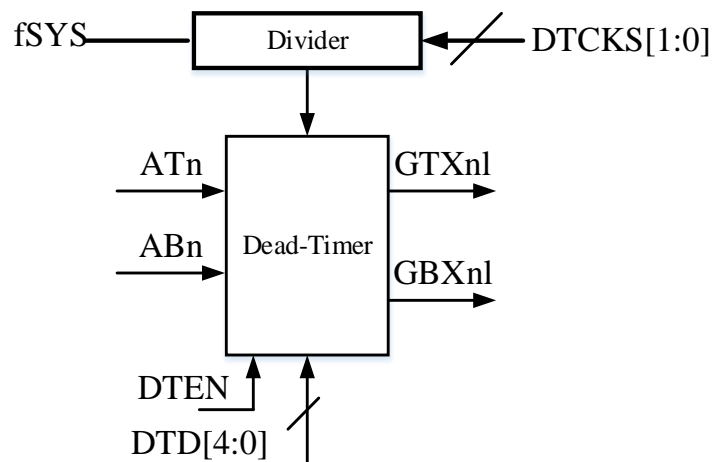
死区时间方框图 (n=0 代表 H 桥左臂，n=1 代表 H 桥右臂)
